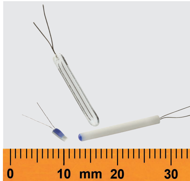
Abb. links: Dünnschicht-Messwiderstand
